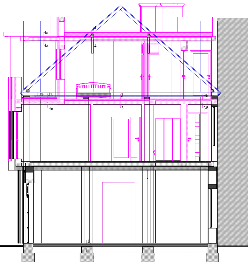
ПРЕСЕК 2-2
