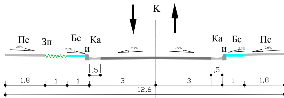
ПРОФИЛ 2-2
