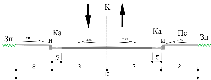
ПРОФИЛ 3-3
