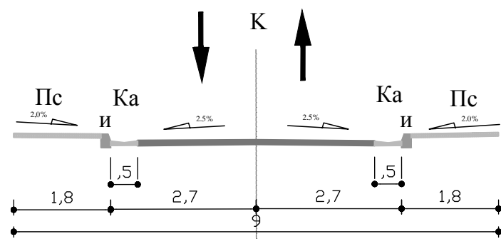
ПРОФИЛ 1-1
