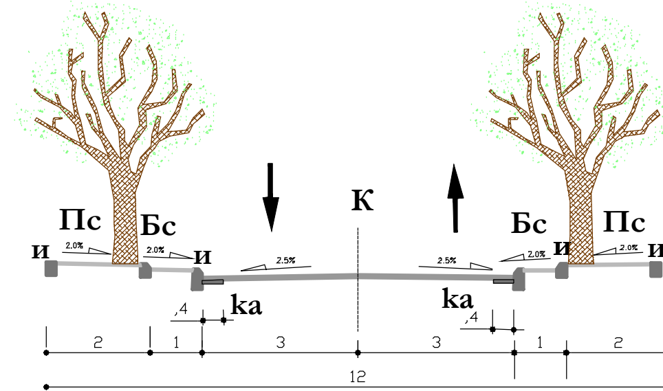
ПРОФИЛ 2-2
