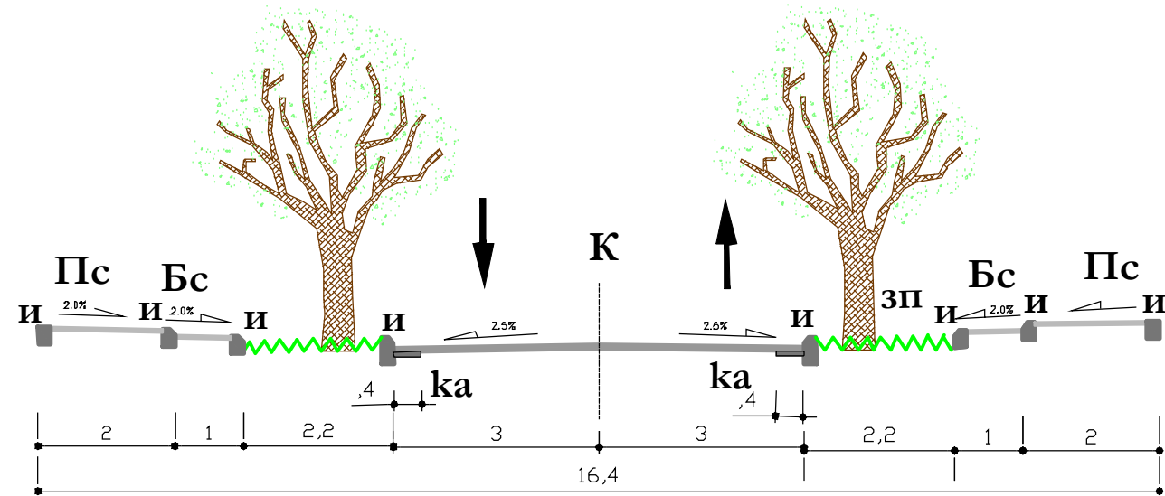
ПРОФИЛ 3-3
