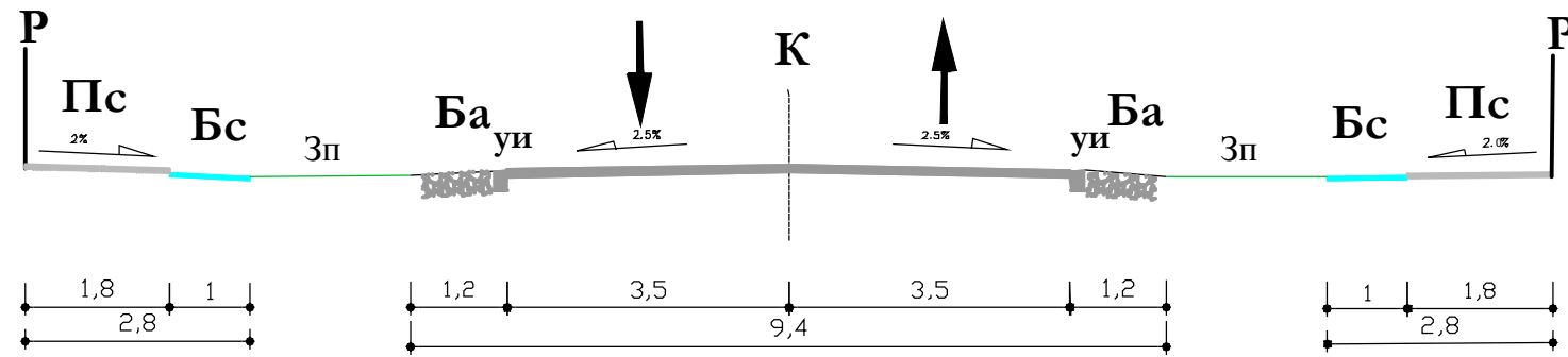
ПРОФИЛ 3-3
